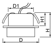
Подсветка для мебели Материал рассеивателя – поликарбонат. Материал корпуса – алюминий.
